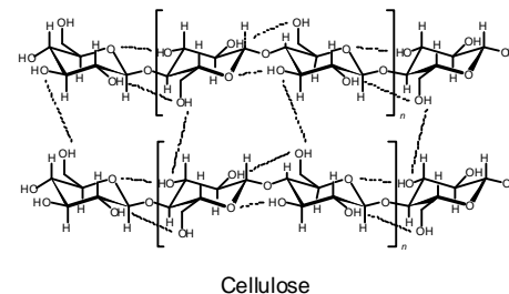
図 デンプン（アミロース）とセルロースの構造式
